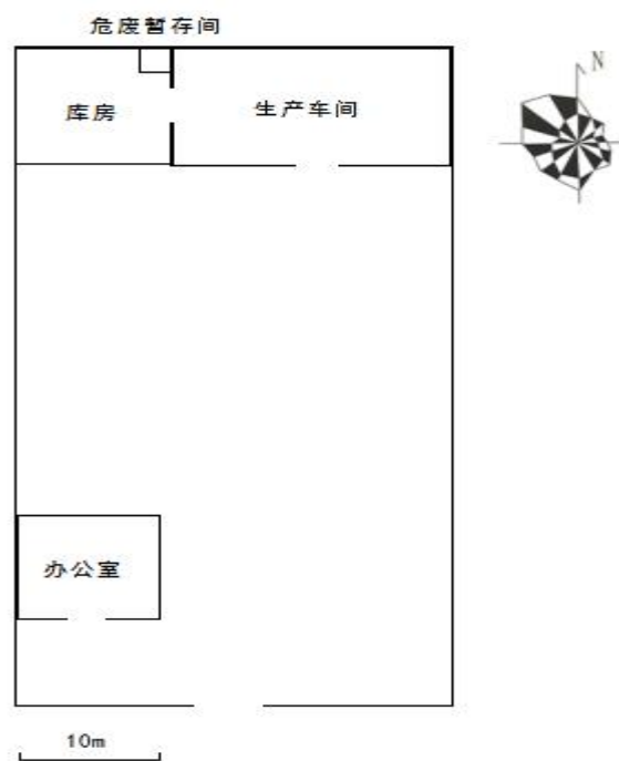
图 2-3 本项目平面布置图
